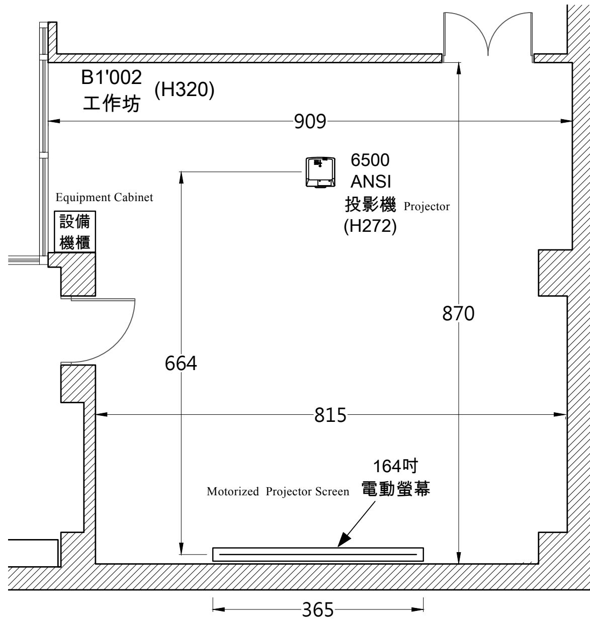
圖 (二) 臺音館工作坊_空間尺寸及視訊配置圖 (單位：公分) Figure(2) Workshop_Floor Plan and Video Plan (Unit: cm)
